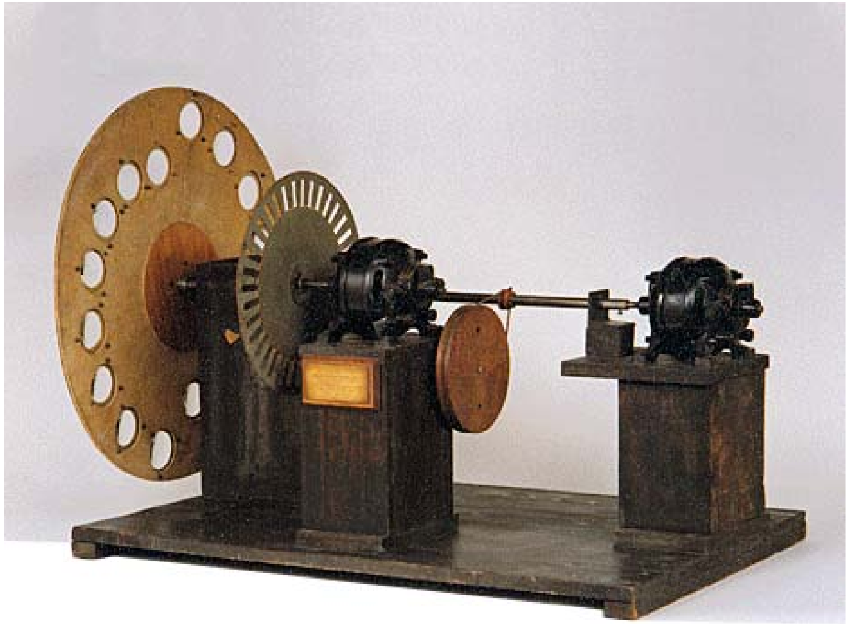
Télévision - émetteur - John Baird - 1926
